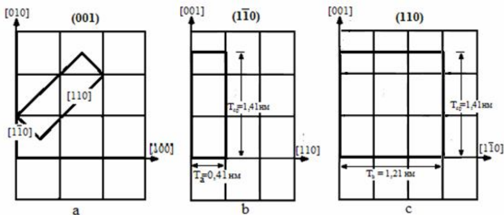
Рис. 3. Схематическое изображение сопряжения периодов идентичности слоев МПС и сверхструктурно упорядоченной области в плоскости подложки (а) и в перпендикулярных к нему плоскостях (б и с).
