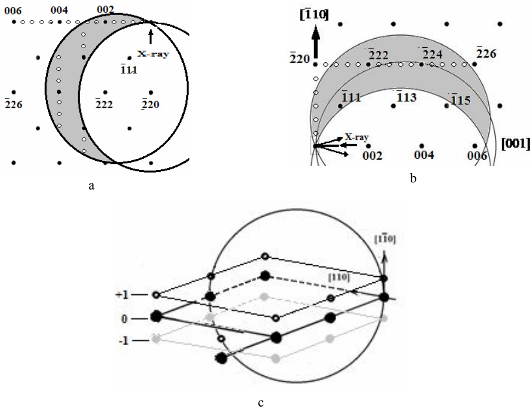
Рис. 2. Схематическое представление метода качания с помощью сферы Эвальда.
