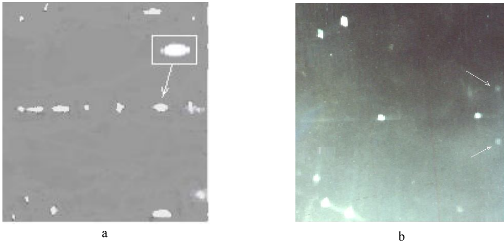
Рис. 1. Фрагменты рентгенограмм качания образца многослойных GaAs/ZnSe со стороны МПС, когда ось качания соответствовала направлениям [110] (a) и [\bar{1}10] подложки (b).
