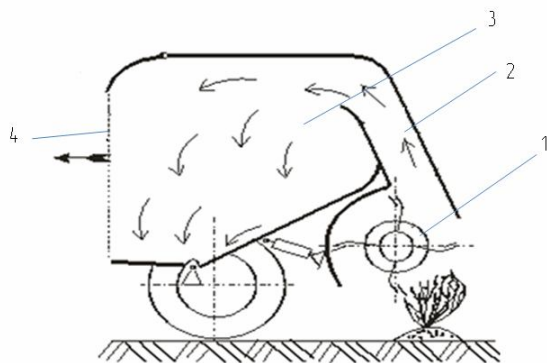
Рис. 3. Схема предлагаемой пустынной косилки-копнителя КПП-3,0: 1 - роторный режущий аппарат, 2 - дефлектор, 3 - бункер, 4 - сетчатая задняя стенка бункера.
